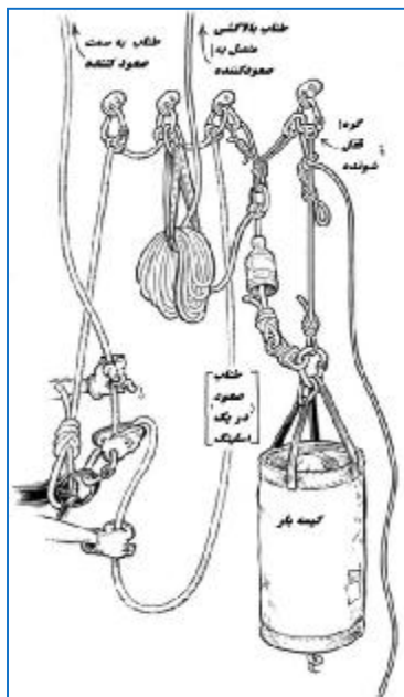
نمونه ای از سازماندهی لیدلاین و تگ لاین (در اینجا صعود با استفاده از تک طناب انجام شده است)
